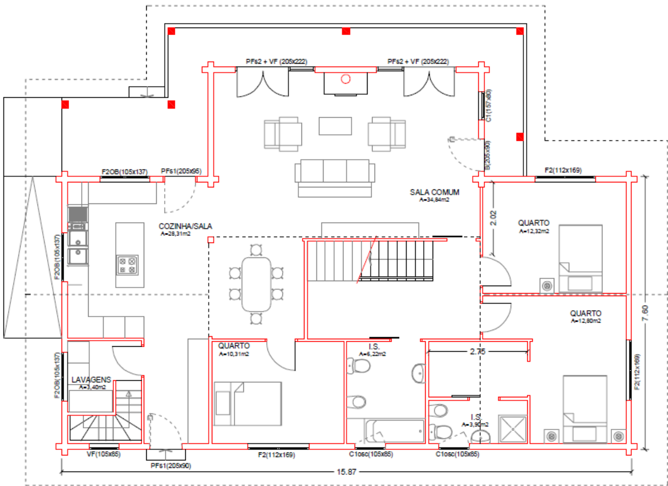
PLANTA DO RDC
