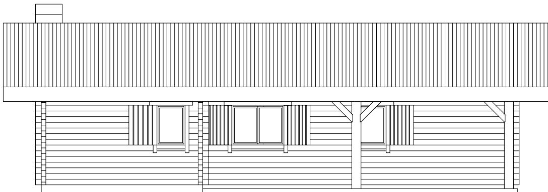
Alçado posterior
