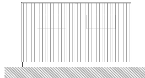
Alçado Posterior
