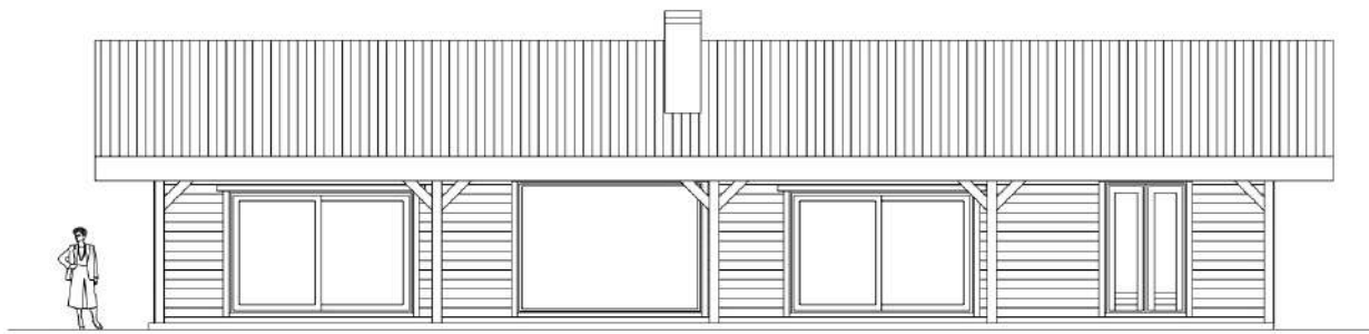
ALÇADO POSTERIOR
