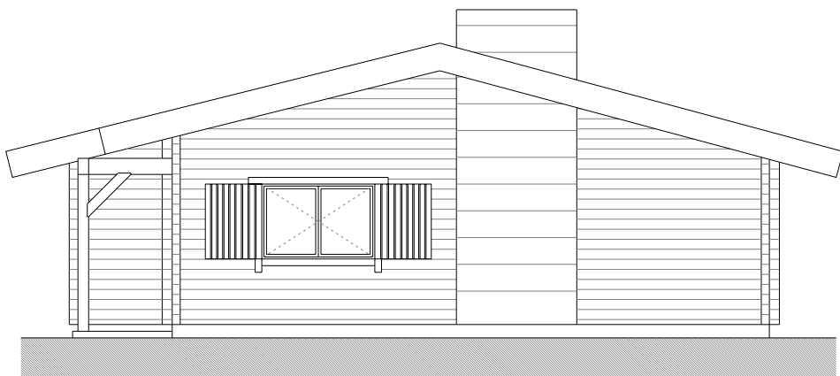
Alçado lateral esquerdo
