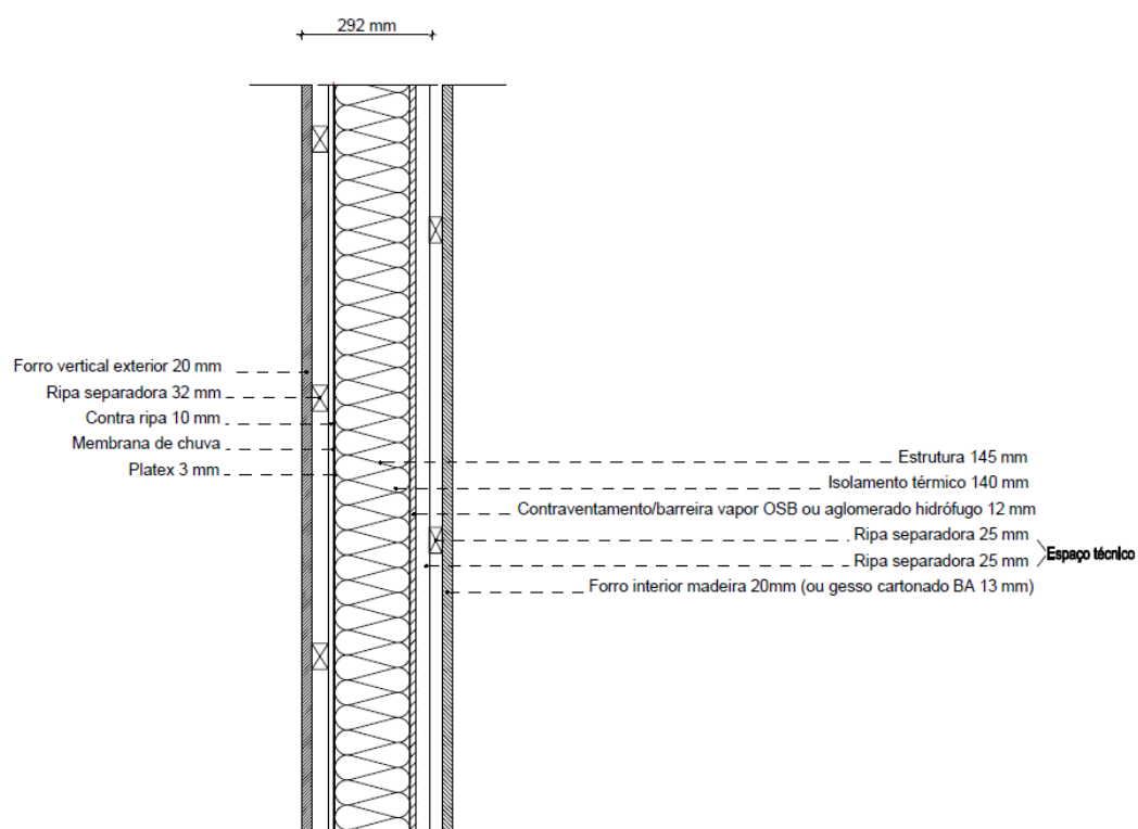
Figura 4: Detalhes construtivos do painel de parede TFS 145: a) corte vertical; b) corte horizontal.
