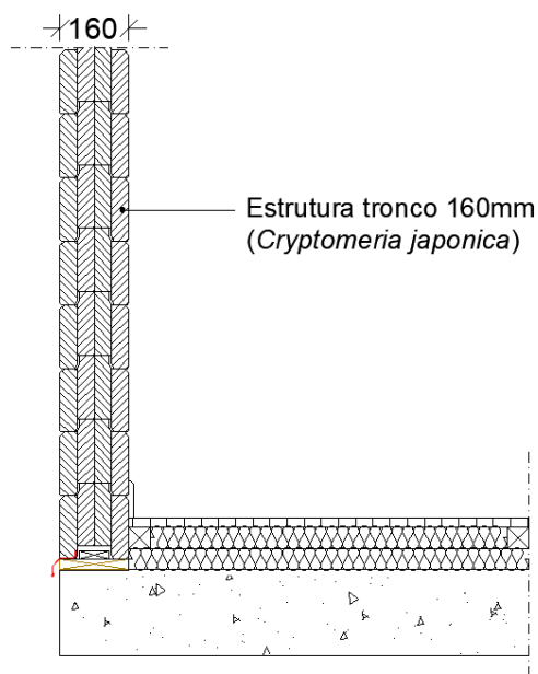
Figura 1: Características geométricas do sistema de fachada “Laminated Timber System – LTS 160”. Vista em corte (dimensões em mm).
