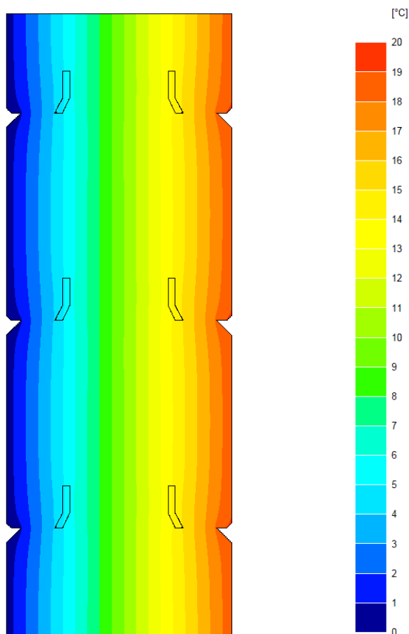
Figura 2: Distribuição bidimensional de temperaturas no sistema de fachada “Laminated Timber System – LTS 160”.
