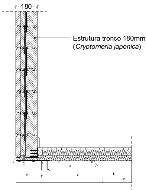
Figura 1: Características geométricas do sistema de fachada “Laminated Timber System – LTS 180”. Vista em corte (dimensões em mm).
