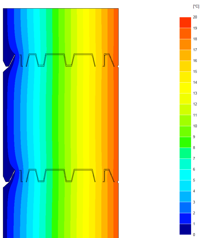
Figura 2: Distribuição bidimensional de temperaturas no sistema de fachada “Laminated Timber System – LTS 180”.
